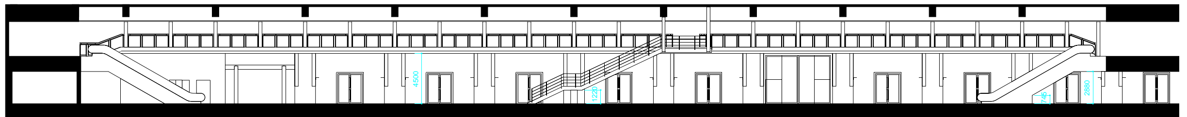
ホワイエ断面図
