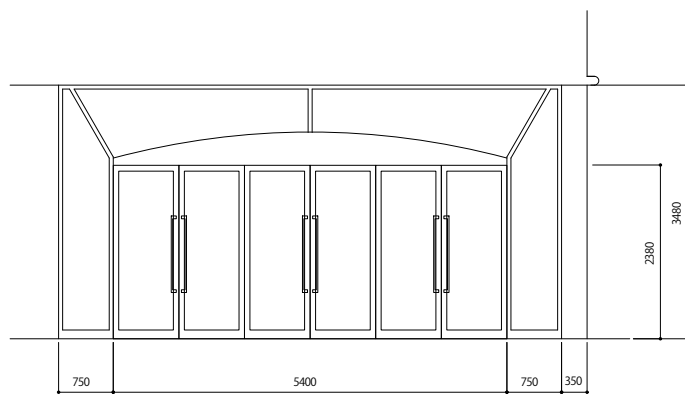
ATCホールエントランス正面図 1/5
