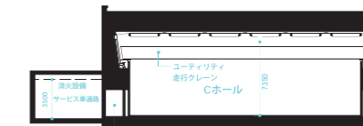
Cホール断面図
