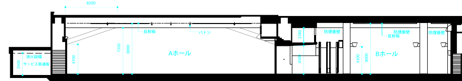
A・Bホール断面図
